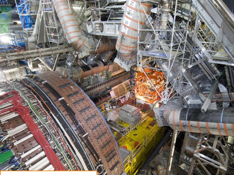
ATLAS detector
